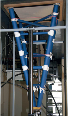
Siegerturm vor dem Abdrücken und Stabilitätsverlust durch das Knicken einer Turmsäule
